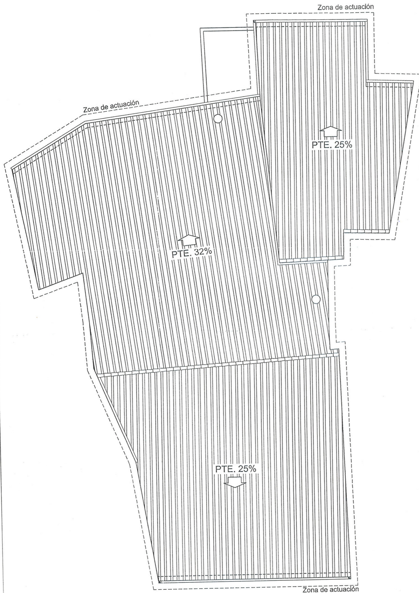
PLANTA CUBIERTA
