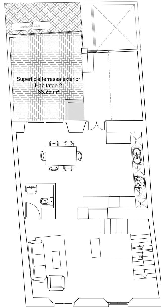
HABITATGE 2 PLANTA SEGONA Sup. útil = 50,10 m 2 Sup. construïda = 69,12 m 2
